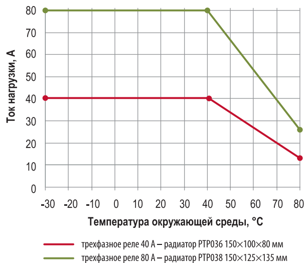
Трехфазное реле с радиатором
