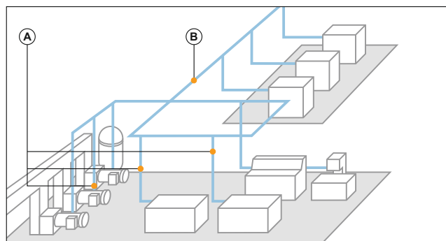
(А) Установка в подводящую трубу для контроля машины. (В) Установка в для контроля нескольких машин.
