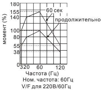
Асинхронный двигатель
