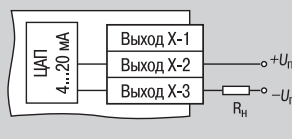
Выходной элемент типа И (ЦАП 4...20 мА)
