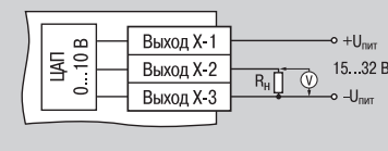
Выходной элемент типа У (ЦАП 0...10 В)
