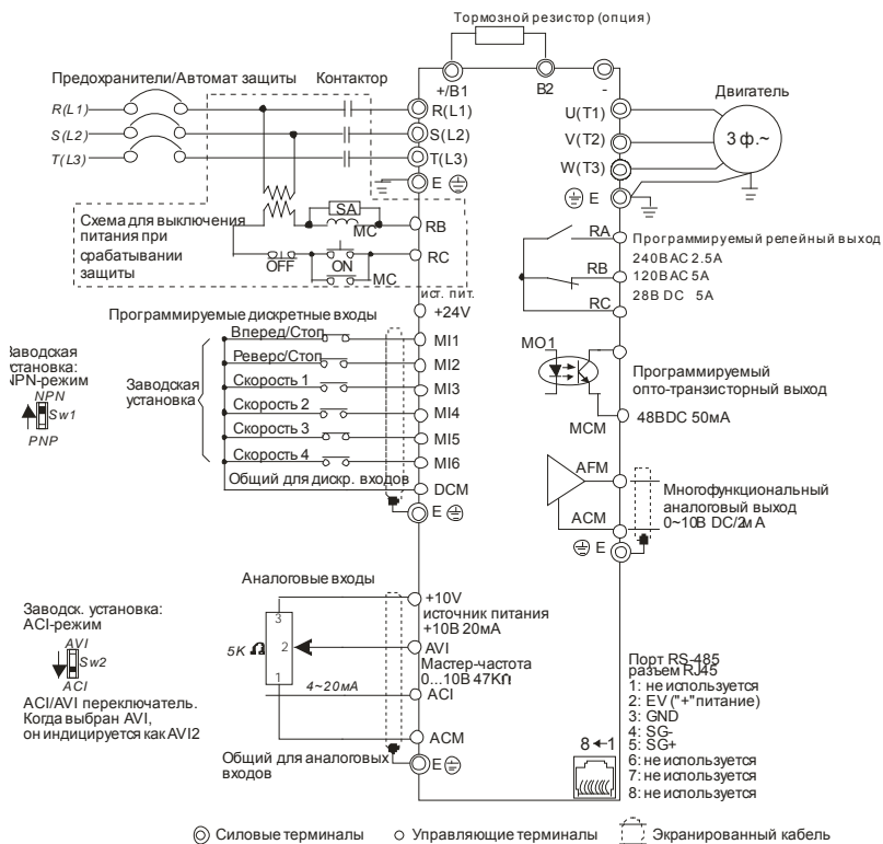
Рисунок 4. Схема для моделей VFD02E23A/43A, VFD037E23A/43A, VFD055E23A/43A, VFD075E23A/43A, VFD110E23A/43A, VFD022E23C/43C, VFD037E23C/43C, VFD055E23C/43C, VFD075E23C/43C, VFD110E23C/43C, VFD150E23A/23C, VFD150E43A/43C, VFD185E43A/43C, VFD220E43A/43C
