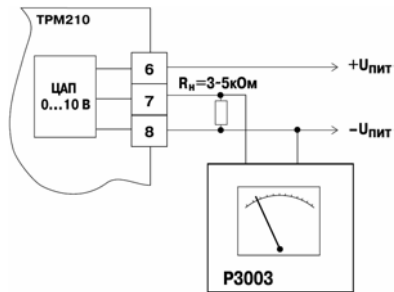
Рисунок Ж.7 – Подключение ВУ2 типа У
