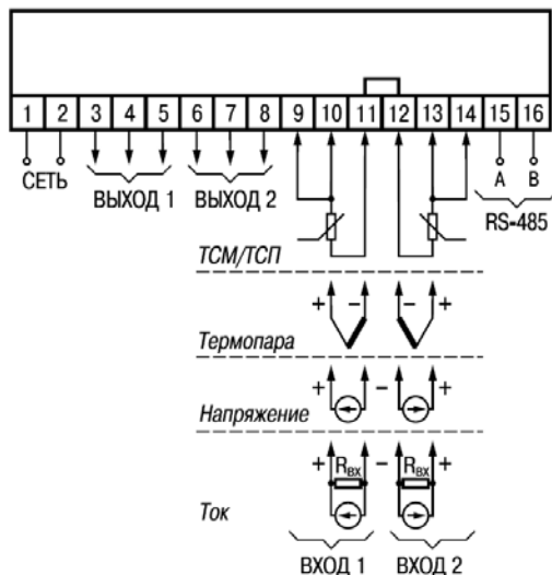
Рисунок В.1 – Общая схема подключения TPM202
