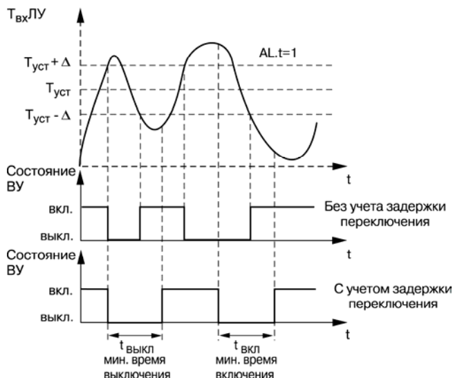
Рис. 3.11. Работа ЛУ с заданным временем удержания
