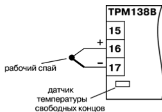
Рис. 3.3. Схема подключения ТП
