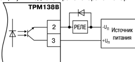
Рис. 3.14. Использование транзисторной оптопары для управления реле
