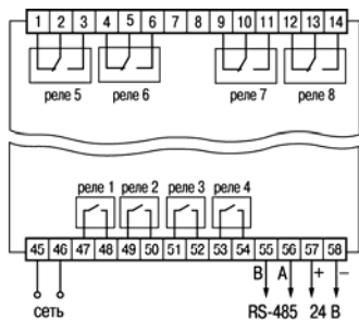
Рис. Б.2. Схема размещения электромагнитных реле в приборе модификации ТРМ 138В-Р
