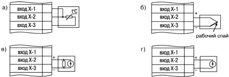
Рис. Б.7. Схемы подключения измерительных датчиков:
