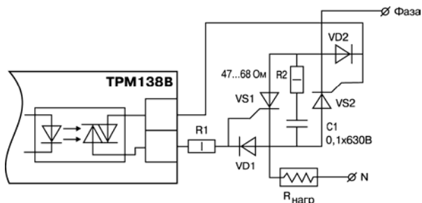
Рис. 3.16. Использование симисторной оптопары для управления силовыми тиристорами
