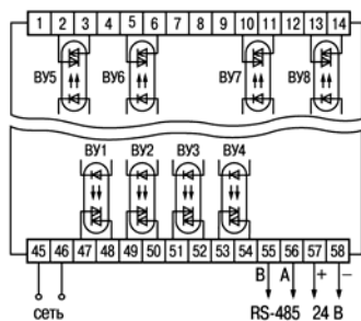
Рис. Б.4. Схема размещения сисмисторных оптопар в приборе модификации ТРМ 138В-С
