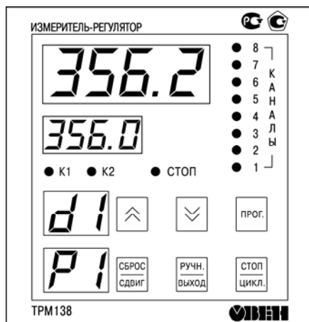
Рис. 3.18. Лицевая панель прибора
