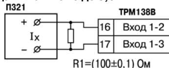
Рис. Д.6. Схема подключения магазина сопротивлений при юстировке
