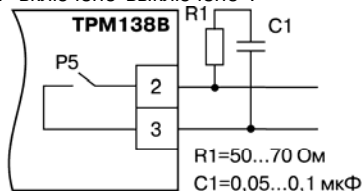
Рис. 3.13. Шунтирование контактов реле при работе с индуктивными нагрузками
