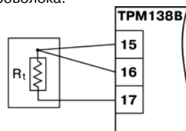
Рис. 3.2. Схема подключения ТС
