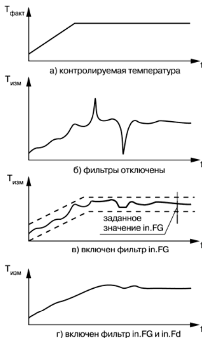
Рис. 3.5. Временные диаграммы работы цифровых фильтров
