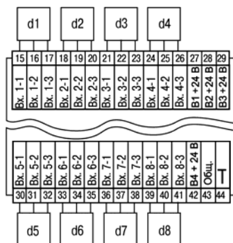
Рис. Б.6. Общая схема подключения измерительных датчиков
