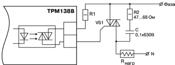
Рис. 3.15. Использование симисторной оптопары для управления силовым симистором
