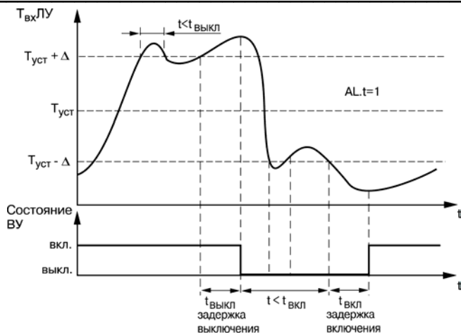
Рис. 3.10. Работа ЛУ с задержками включения и выключения
