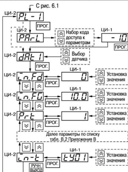
Рис. 7.3. Схема установки программируемых параметров на уровне PL-1
