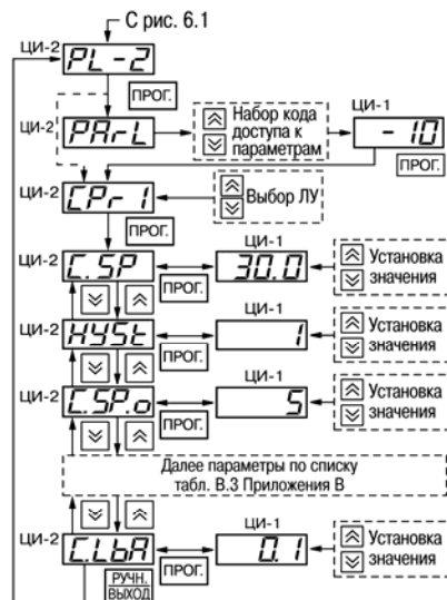
Рис. 7.4. Схема установки программируемых параметров на уровне PL-2
