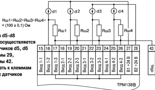
Рис. Б.8. Пример схемы подключения активных датчиков d1 - d4
