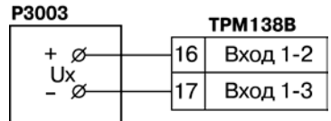
Рис. Д.5. Схема подключения компаратора напряжения при юстировке
