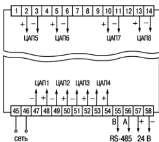
Рис. Б.5. Схема размещения ЦАП в приборе модификации ТРМ 138В-И
