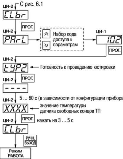
Рис. Д.4. Схема проведения юстировки датчика свободных концов ТП
