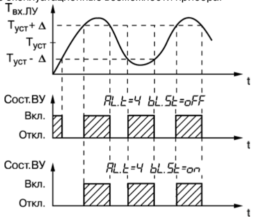
Рис. 3.9. Диаграммы работы ЛУ при различном значении bL.St
