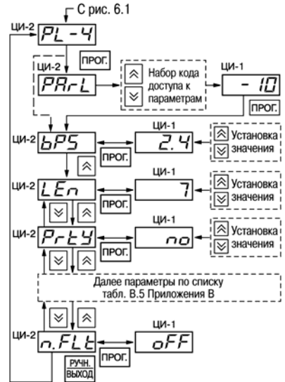
Рис. 7.6. Схема установки программируемых параметров на уровне PL-4
