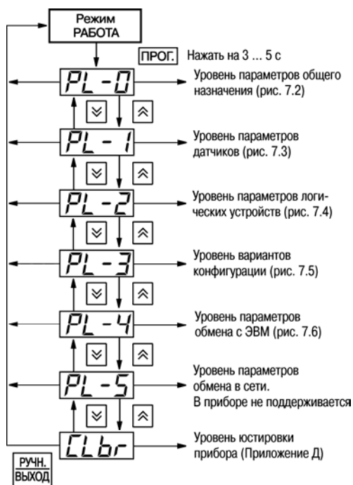
Рис. 6.1. Схемы выбора уровня программируемых параметров
