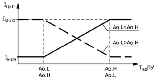
Рис. 3.12. Выходные характеристики ЦАП
