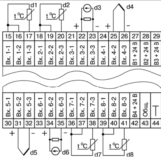
Рис. Б.10. Пример подключения датчиков различного типа
