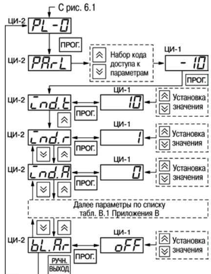
Рис. 7.2. Схема установки программируемых параметров на уровне PL-0
