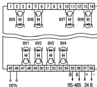
Рис. Б.3. Схема размещения транзисторных оптопар в приборе модификации ТРМ 138В-К
