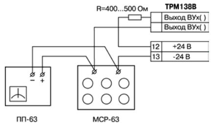
Рис. Д.7. Схема подключения аппаратуры при юстировке ЦАП
