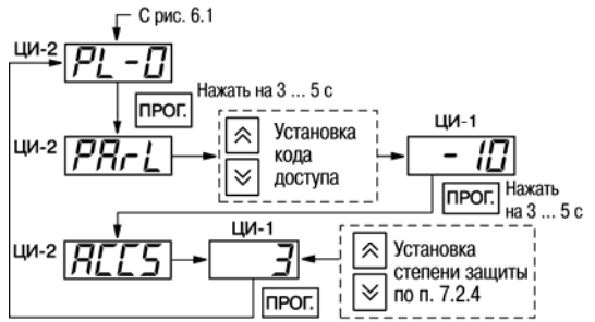
Рис. 7.1. Схемы установки степени защиты
