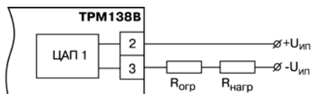
Рис. 3.17. Схема соединения ЦАП с нагрузкой
