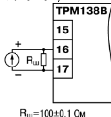
Рис. 3.4. Схема подключения датчика с токовым выходом
