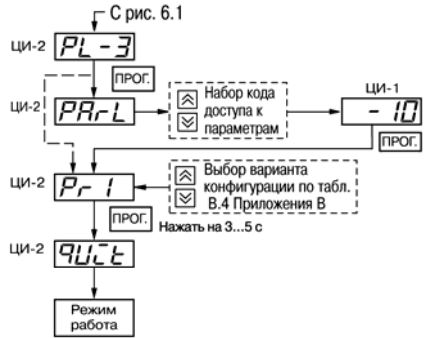
Рис. 7.5. Схема выбора конфигурации на уровне PL-3
