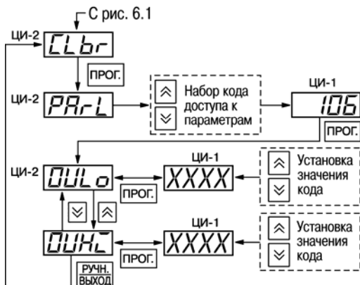
Рис. Д.8. Схема проведения юстировки ЦАП
