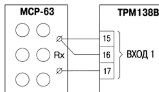
Рис. Д.1. Схема подключения магазина сопротивлений при юстировке
