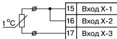
Рис. Г. 1. Схема подключения термометра сопротивления по двухпроводной схеме
