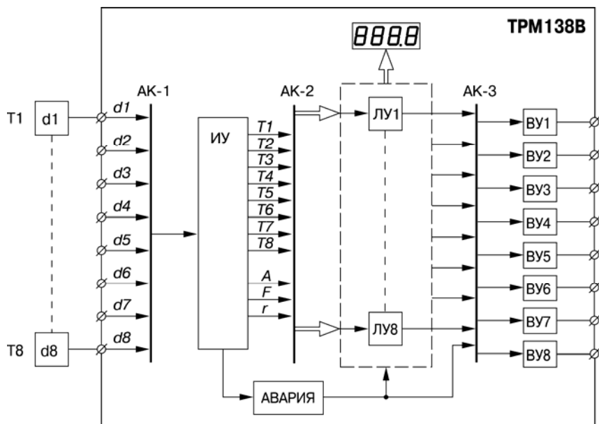
Рис. 3.1. Функциональная схема прибора
