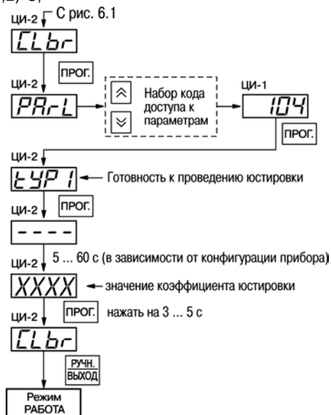
Рис. Д.2. Схема проведения юстировки прибора для работы с первичным преобразователем
