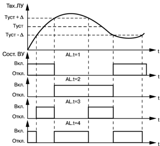
Рис. 3.8. Выходные характеристики компараторов
