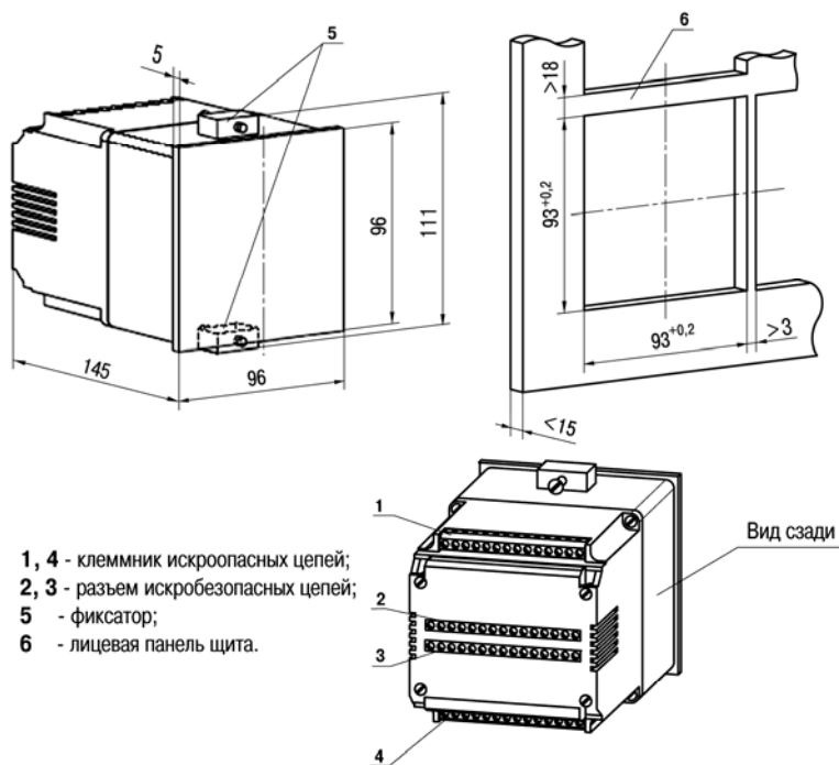
Рис. А. 1. Габаритный чертеж TPM138В
