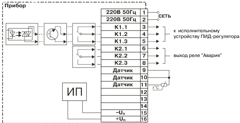
Рисунок Е.1. Схема подключения к прибору TRM10X термопреобразователя сопротивления (для конструктивного исполнения "Н", "Щ1" и "Щ2")
