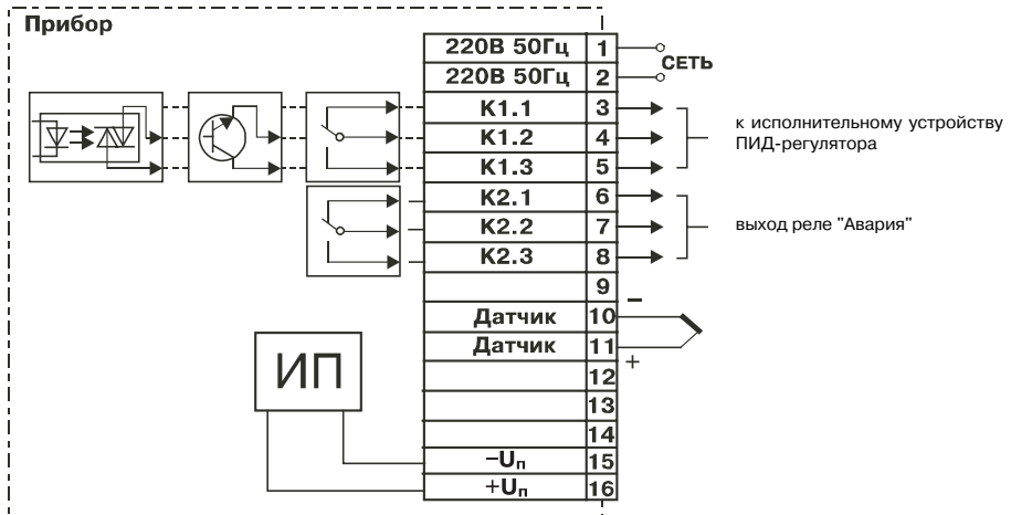
Рисунок Е.2. Схема подключения к приборам TRM10X терморпар (для конструктивного исполнения "Н", "Щ1" и "Щ2")
