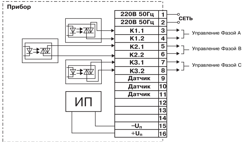
Рисунок Е.4. Схема подключения прибора ТРМ10Х-Х.Х.С3, используемого для управления устройствами с трехфазной нагрузкой
