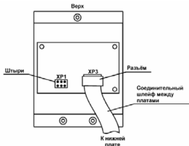
Рис. 5. Расположение коммутатора XR1. Вид обратной стороны передней платы монитора при снятой крышке
