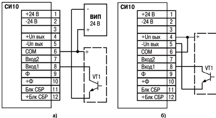
Рисунок Б.3 – Подключение активных датчиков, имеющих на выходе транзистор n-p-n типа с открытым коллекторным входом: а) при работе от внешнего источника питания; б) при работе от питающего напряжения прибора
