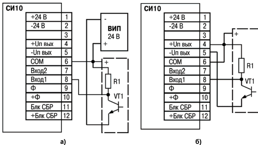
Рисунок Б.2 – Подключение пассивных датчиков, имеющих на выходе транзистор n-p-n типа с открытым коллекторным входом:
