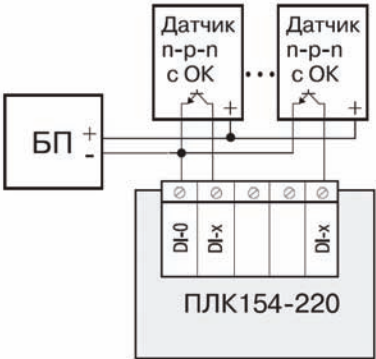
Рис. Б6. Схема подключения к ПЛК154 дискретных датчиков с полупроводниковым выходным каскадом
