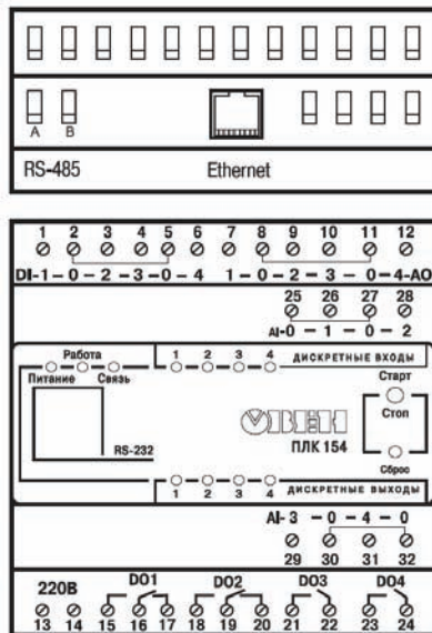
Рис. 1. Внешний вид ПЛК154
