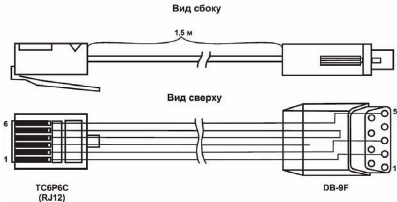
Рис. Б3. Схема кабеля программирования, входящего в комплект поставки
