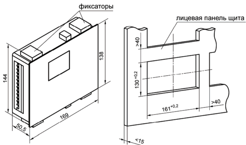
Рисунок А.2 – Габаритный чертёж прибора в корпусе Щ7
