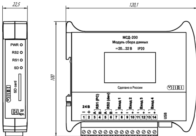
Рисунок А.1 – Габаритный чертёж модуля
