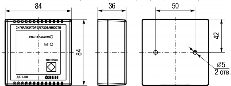
Рисунок 3.1 – Габаритные и установочные размеры прибора
