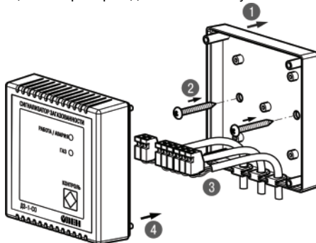
Рисунок 5.1 – Монтаж прибора
