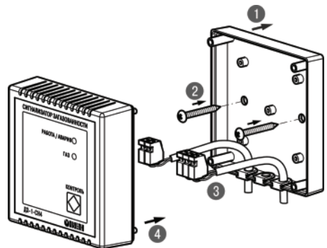
Рисунок 5.1 – Монтаж прибора
