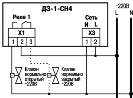
Рисунок 5.3 – Типовая схема подключения прибора
