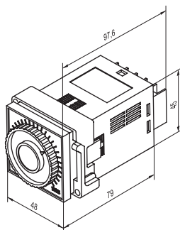
Габаритный чертеж
