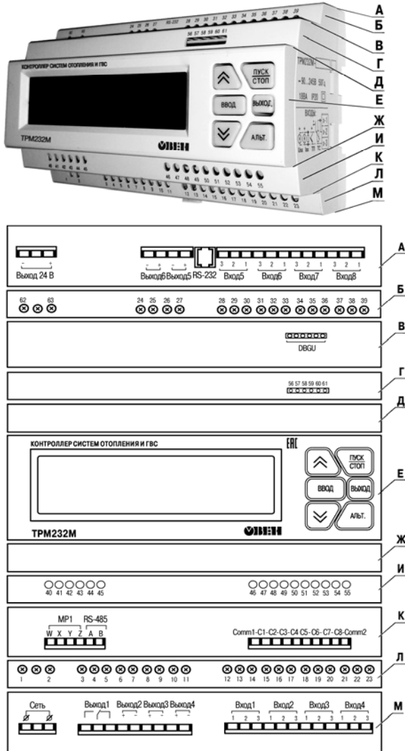
Рисунок 3.1 – Прибор ТРМ232М-01: клеммники, элементы индикации и управления
