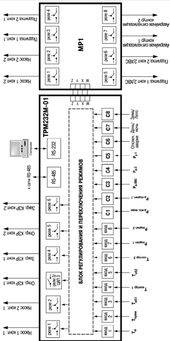
Рисунок 3.9 – Функциональная схема прибора - два контура
