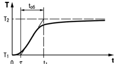
Рисунок Г.2 – График переходной функции
