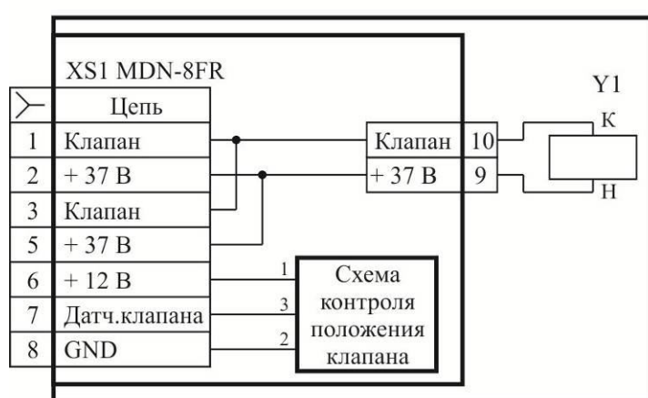
а) с разъемом MDN-8FR
