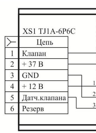
б) с разъемом TJ1A-6P6C
