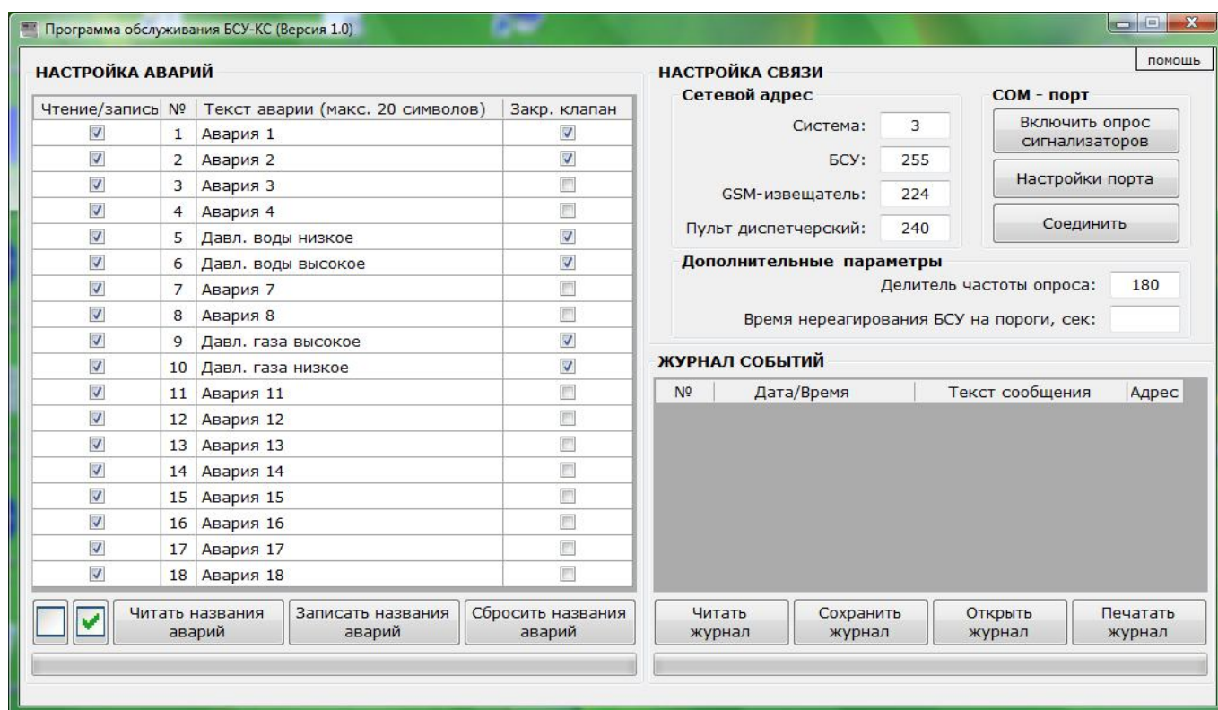
Рисунок 15 – Рабочее окно программы BsuViewer.
