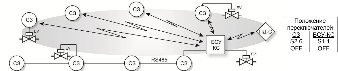
г) индивидуальная с радиоканалом и RS485
