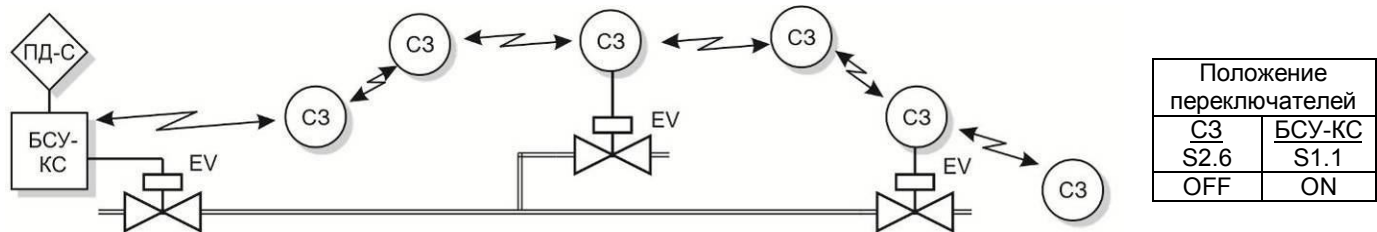
б) линейная с радиоканалом
