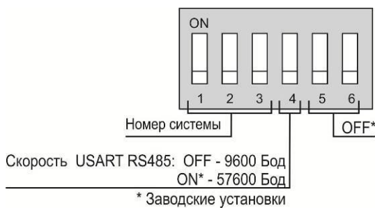
Рисунок 16 – Группа переключателей «Конфигурация»
