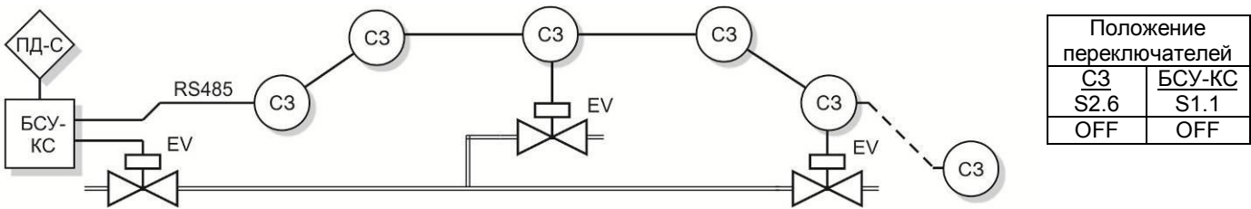
а) индивидуальная с RS485
