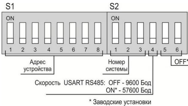
Рисунок 17 – Ретранслятора Р-433. Расположение переключателей.
