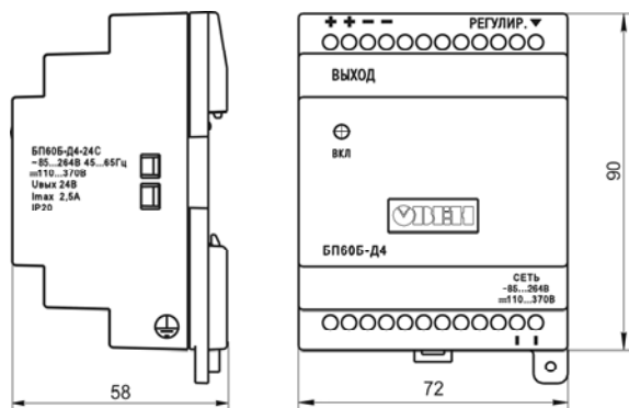
Рисунок 3.1 – Габаритные размеры блока
