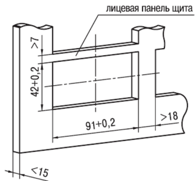
Рисунок А.3 – Прибор щитового крепления в корпусе типа Щ2
