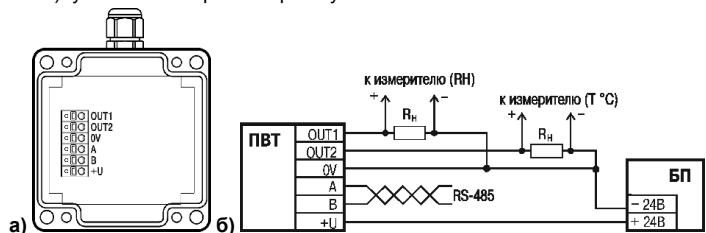
Рисунок 5.1 – Подключение прибора: а) расположение клемм; б) схема электрических соединений
