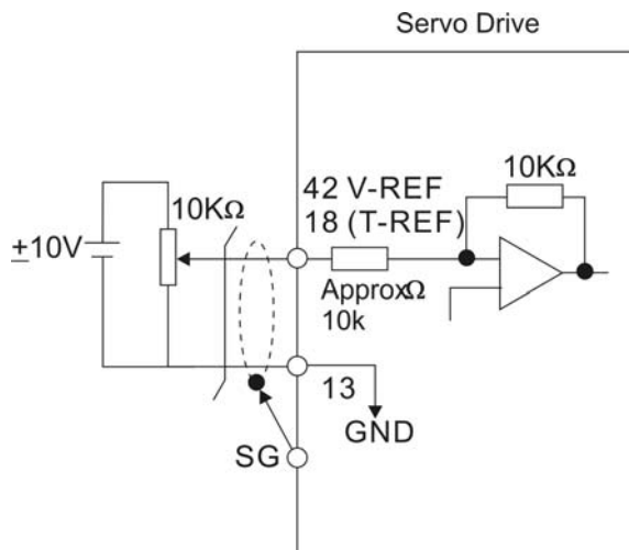
C1: Аналоговое задание скорости / момента
