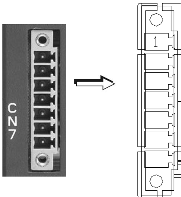
Рис. 3.14. Разъем CN7
