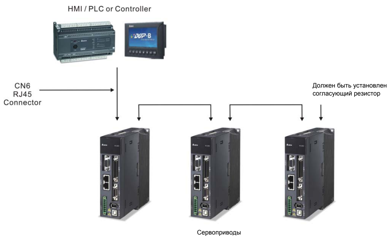
Рис. 3.18. Связь нескольких сервоприводов по CANopen
