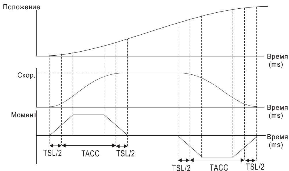
Характеристика движения. Постоянные времени фильтра и ускорения.
