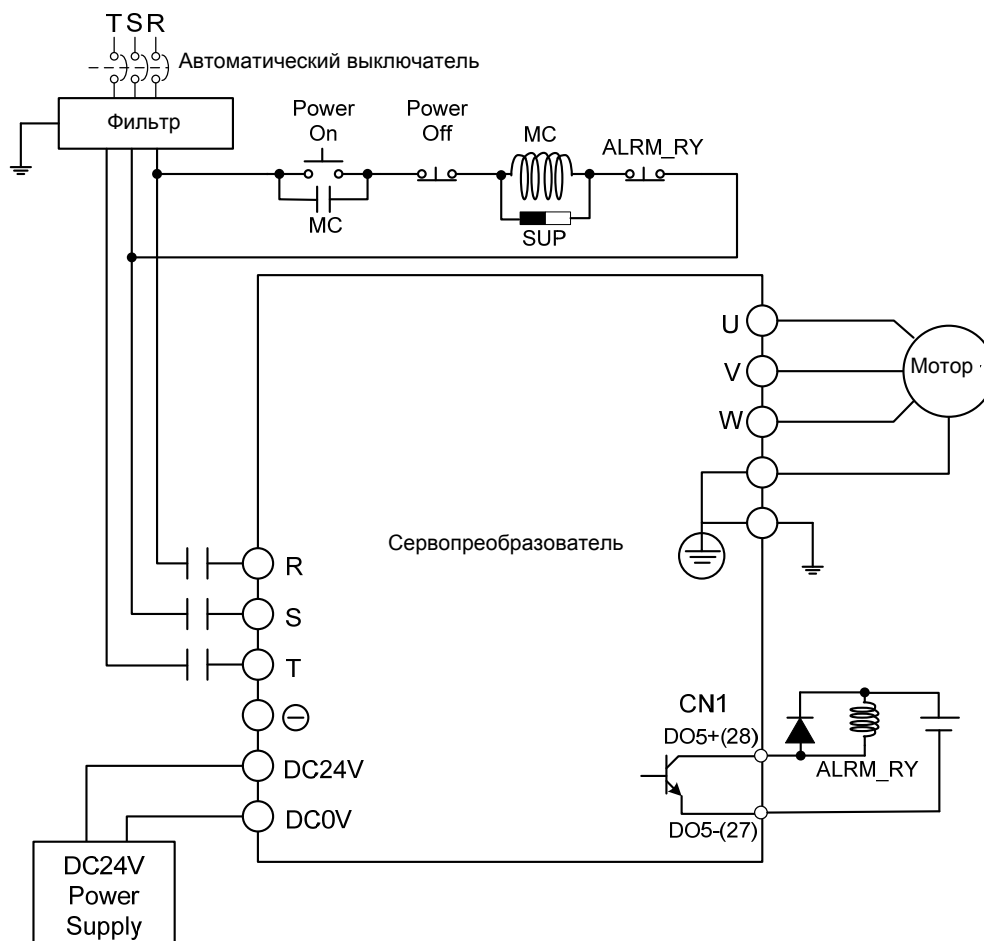
Рис. 3.5. Трехфазный источник питания (для всех моделей)
