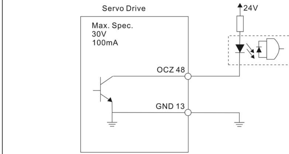
C15: Сигнал энкодера Z (открытый коллектор)
