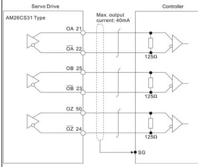
C13: Выходные сигналы энкодера (линейный драйвер)
