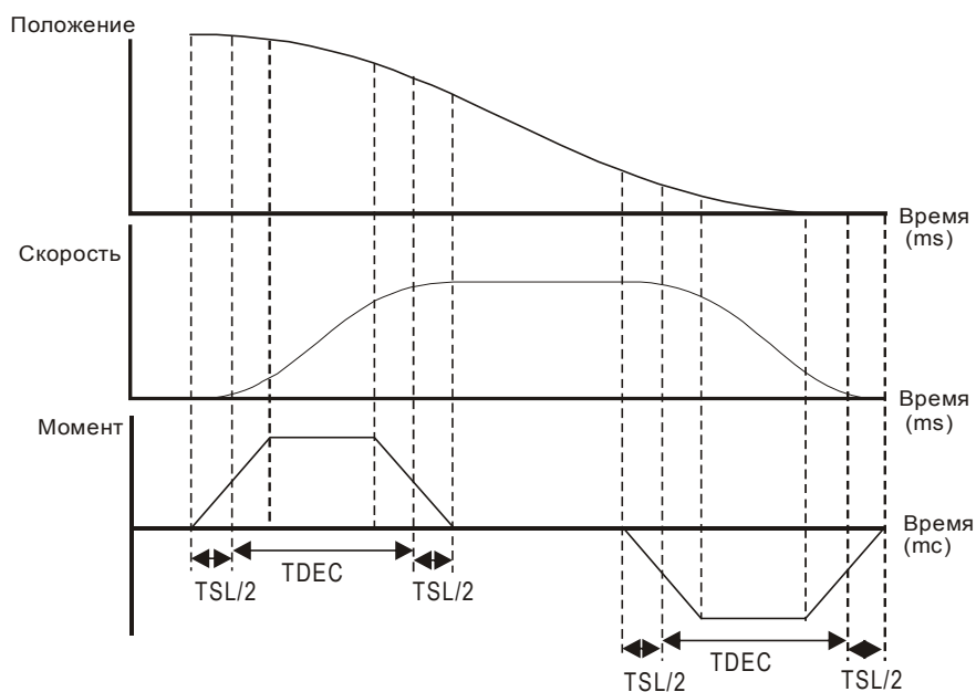
Характеристика движения. Постоянные времени фильтра и замедления.
