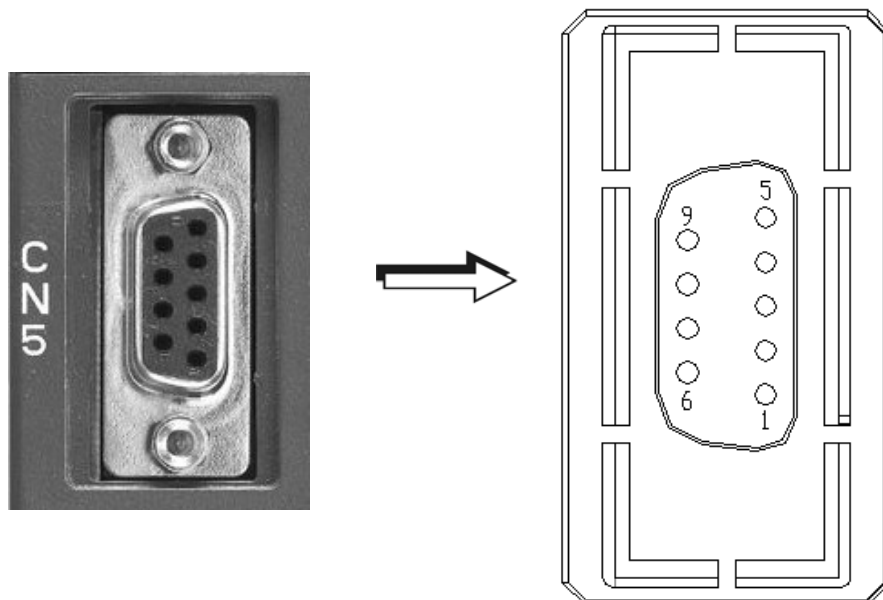
Рис. 3.16. Разъем CN5
