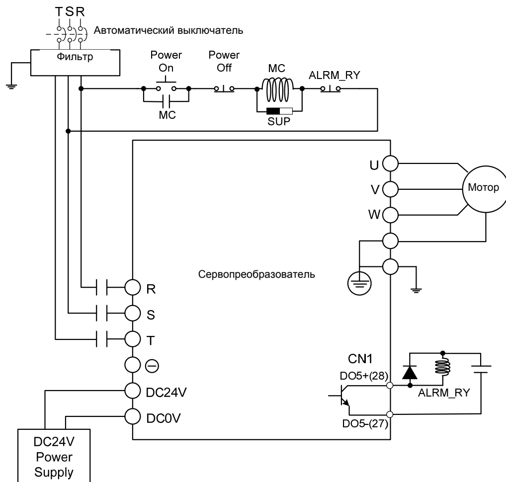
Рис. 3.3. Трехфазный источник питания (для всех моделей)
