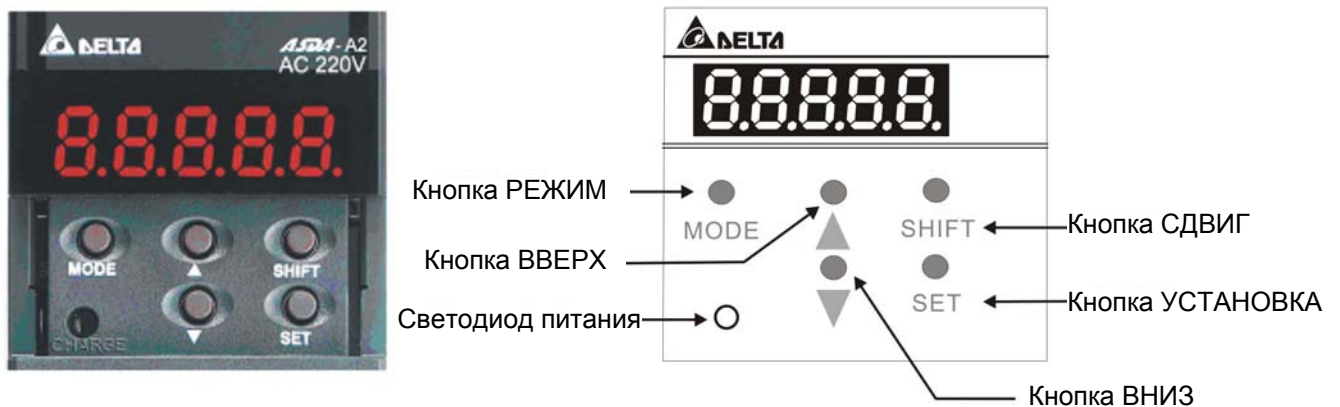
Рис. 4.1. Панель управления
