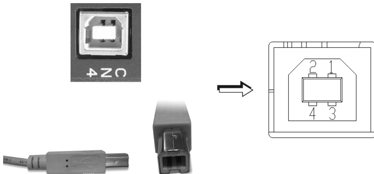
Рис. 3.15. Разъем CN4
