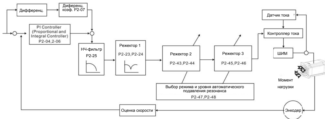
Блок-диаграмма управления скоростью
