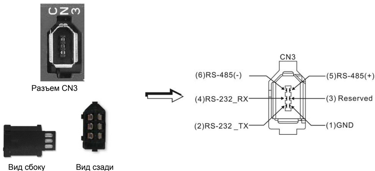
Рис. 3.14. Разъём CN3
