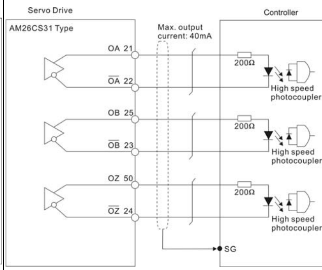
C14: Выходные сигналы энкодера (оптопара)
