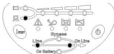
Рис. 4-2 Панель управления в режиме двойного преобразования
