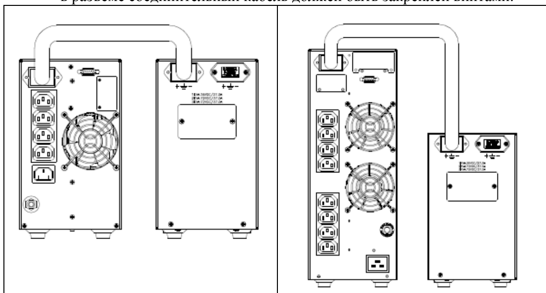
Рис. 3-2.1 ИБП мощностью 1 кВА
