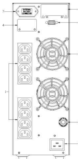
Рис. 2-4 ИБП мощностью 2 кВА и 3 кВА
