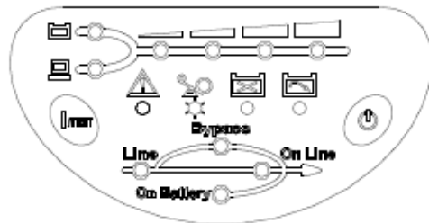
Рис. 4-8 Индикация короткого замыкания на выходе ИБП
