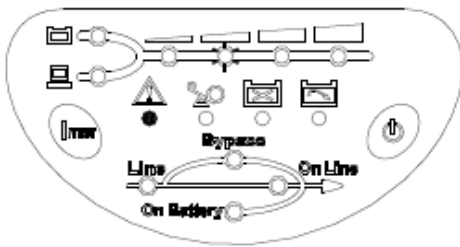
Рис. 4-9 «НЕДОСТАТОЧНОЕ ВЫХОДНОЕ НАПРЯЖЕНИЕ»
