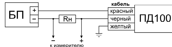
Рис. 1 Схема подключения преобразователя
