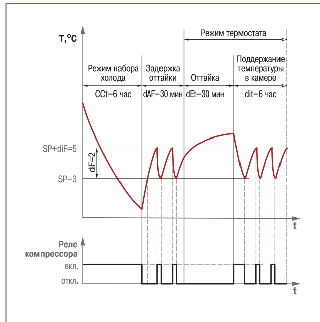
▶ Пример работы TRM974 в режиме НАБОР ХОЛОДА: график изменения температуры в камере и временная диаграмма работы реле компрессора (для значений параметров, установленных по умолчанию на заводе-изготовителе)
