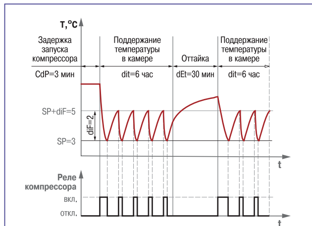
▲ Пример работы TRM961 в режиме ТЕРМОСТАТ: график изменения температуры в камере и временная диаграмма работы реле компрессора (для значений параметров, установленных по умолчанию на заводе-изготовителе)
